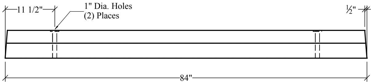
ELEVATION
